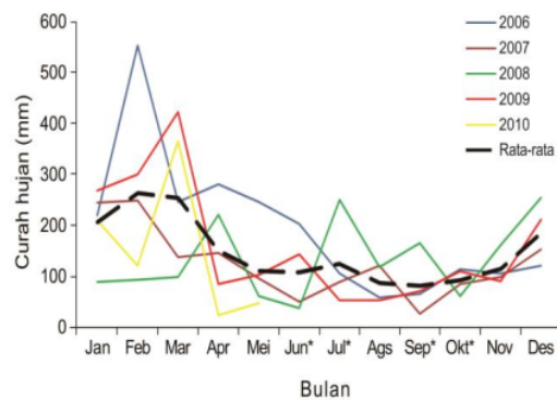
Gambar 2 Data curah hujan Manokwari dan sekitarnya (BMKG 2012).
