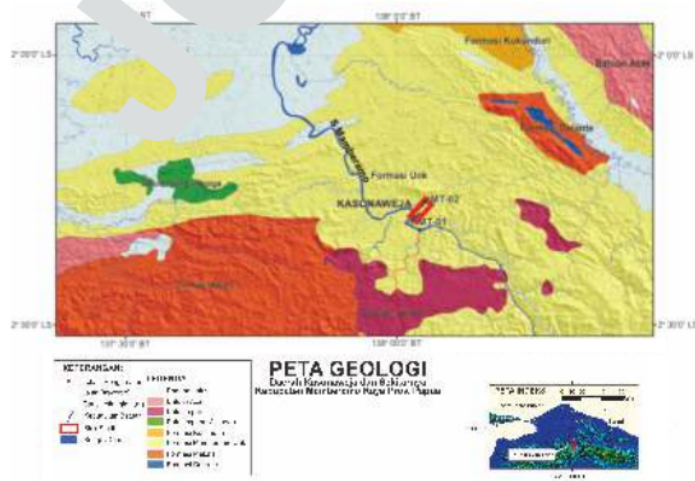
Gambar 2. Peta geologi daerah Mamberamo dan sekitarnya, yang memperlihatkan sebaran Formasi Mamberamo (Modifikasi Gaofer & Budhitrinsa, 1995; dan Hakim dkk,1995;). Poligon merah menunjukan lokasi penelitian.
