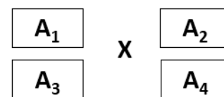
Gambar 1. Desain Penelitian
